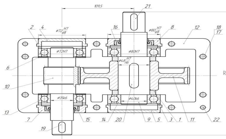
Рисунок 3. Чертеж редуктора.
