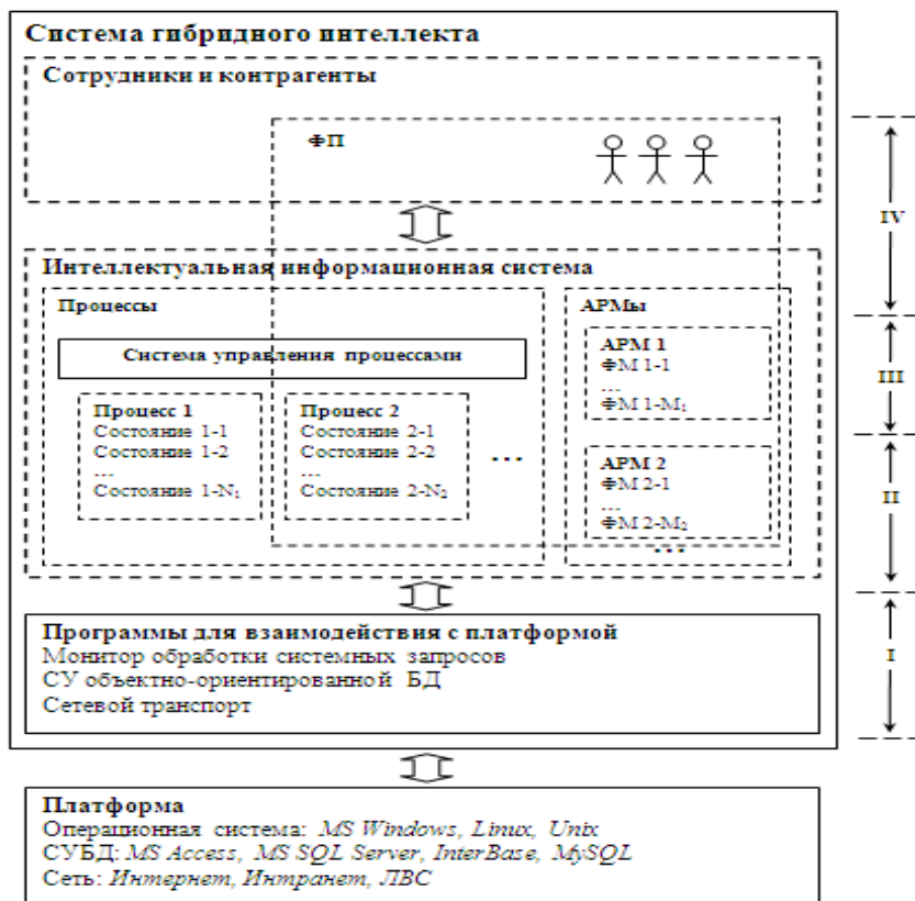
Рисунок 1 – Функционально-структурная схема СГИ
