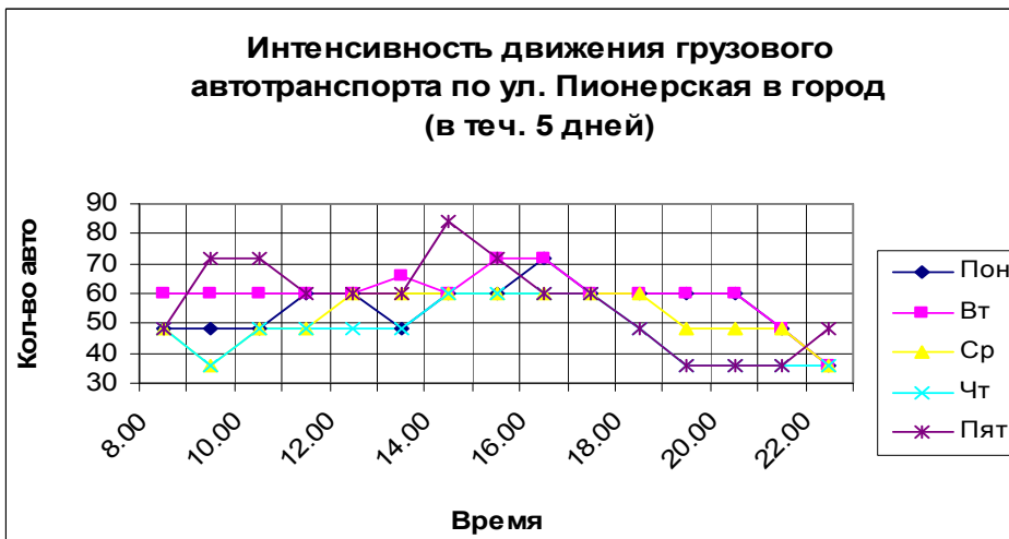
Рисунок 3 – Графическая модель грузового автотранспорта по улице Пионерская в город
