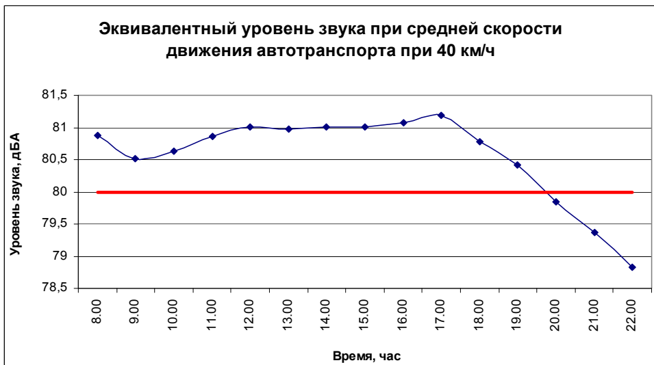
Рисунок 8 – Модель эквивалентного уровня звука легкового автотранспорта при скорости движения 40 км/ч
