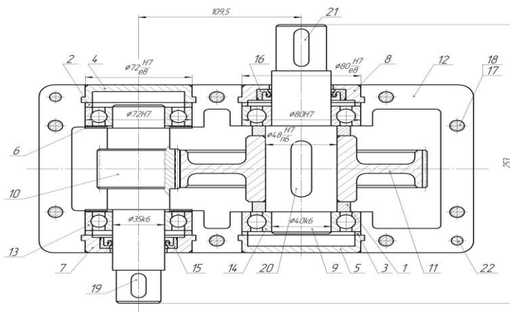
Рисунок 4 – Чертеж редуктора.
